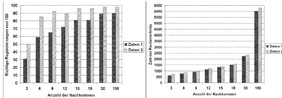
Abb. 3. Variation der Anzahl der Nachkommen ( Var_r = 0.001 , Var_t = 1 und P_u = 1 ), links richtige Registrierungen von 100, rechts die benötigten Rechenschritte.
