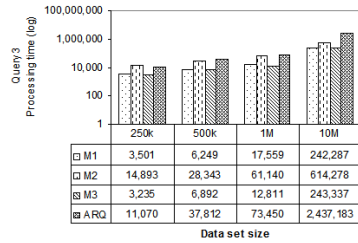
(e) Query3 (BSBM)
