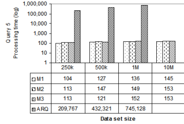
(d) Query5 (SP 2 B)
